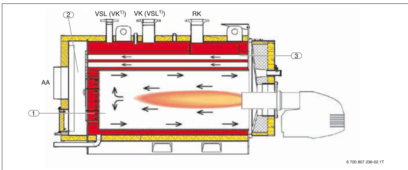
Gráfico 4 Flujo de los gases calientes de combustión en el interior de la caldera Uni 3000 F
