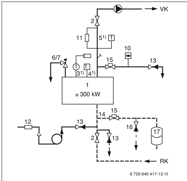
Gráfico 18 Equipamiento de seguridad conforme a la normativa EN 12828 para calderas \geq 300 kW con un limitador de temperatura de seguridad \leq 110^{\circ}\text{C}
