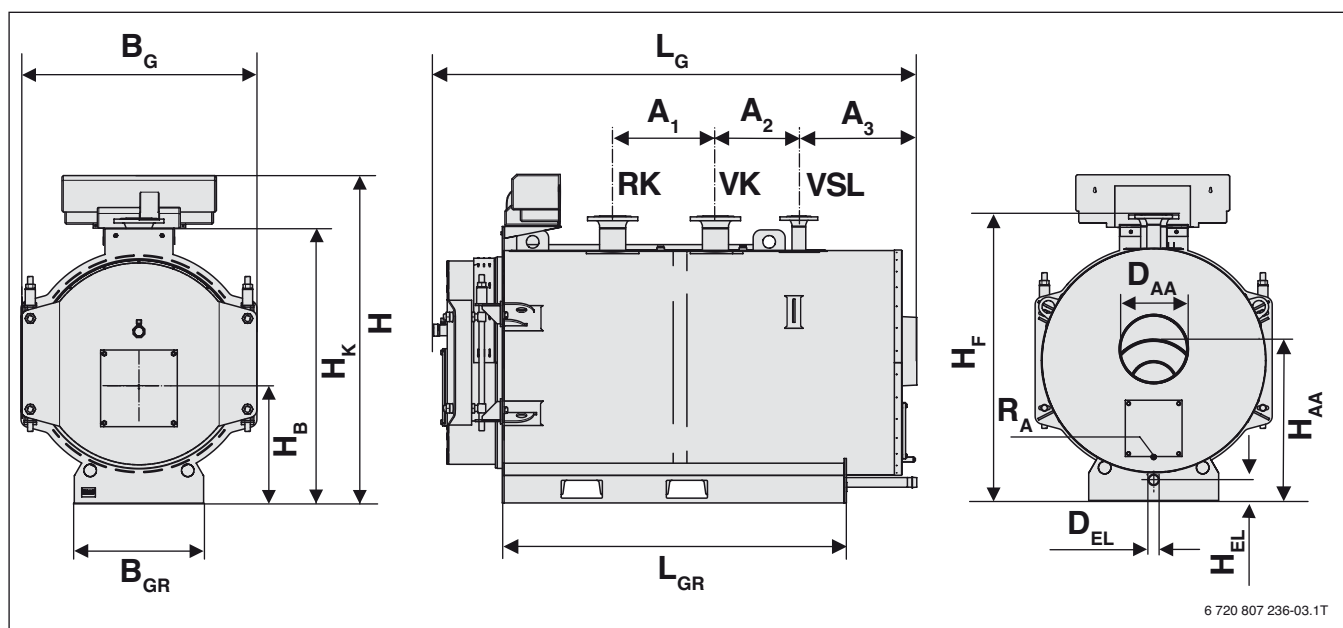
Gráfico 5 Dimensiones, Uni 3000 F (420 kW a 820 kW)
