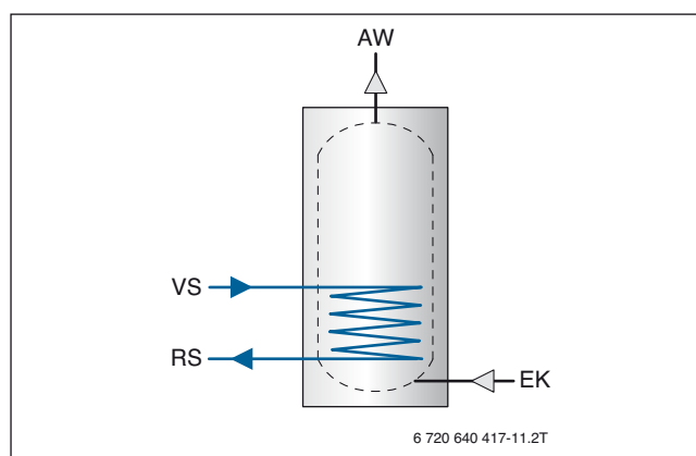
Gráfico 16 Calentamiento de A.C.S. conforme al principio de acumulación con serpentines indirectos internos
