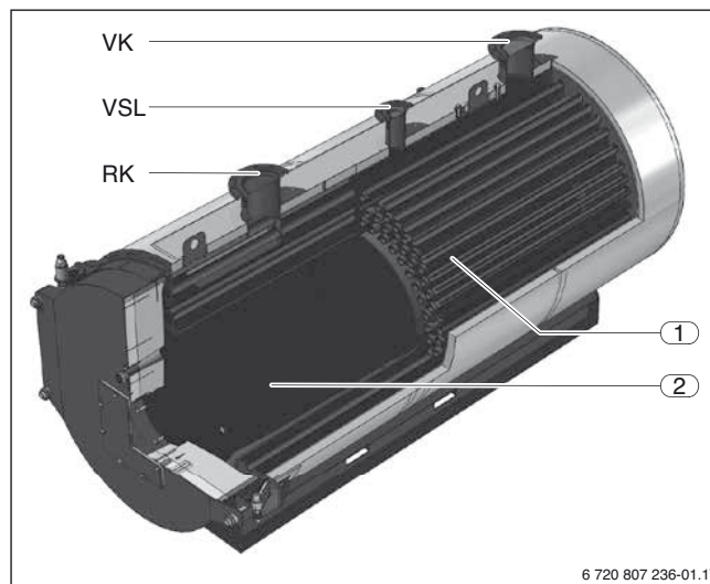
Gráfico 3 Circulación del agua en el interior de la caldera Uni 3000 F
