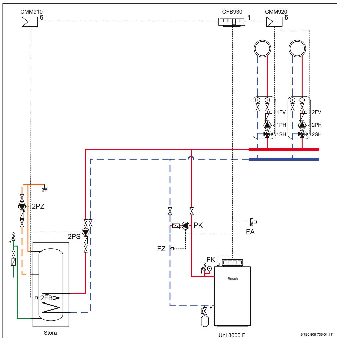
Gráfico 26 Ejemplo de sistema para Uni 3000 F
