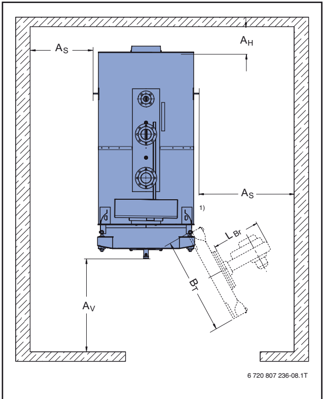
Gráfico 29 Sala para la caldera Uni 3000 F
