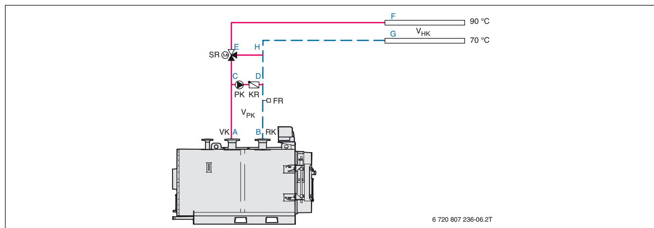
Gráfico 21 Ejemplo de circuito hidráulico para un sistema de una sola caldera con bomba de caldera en el bypass para la caldera Uni 3000 F
