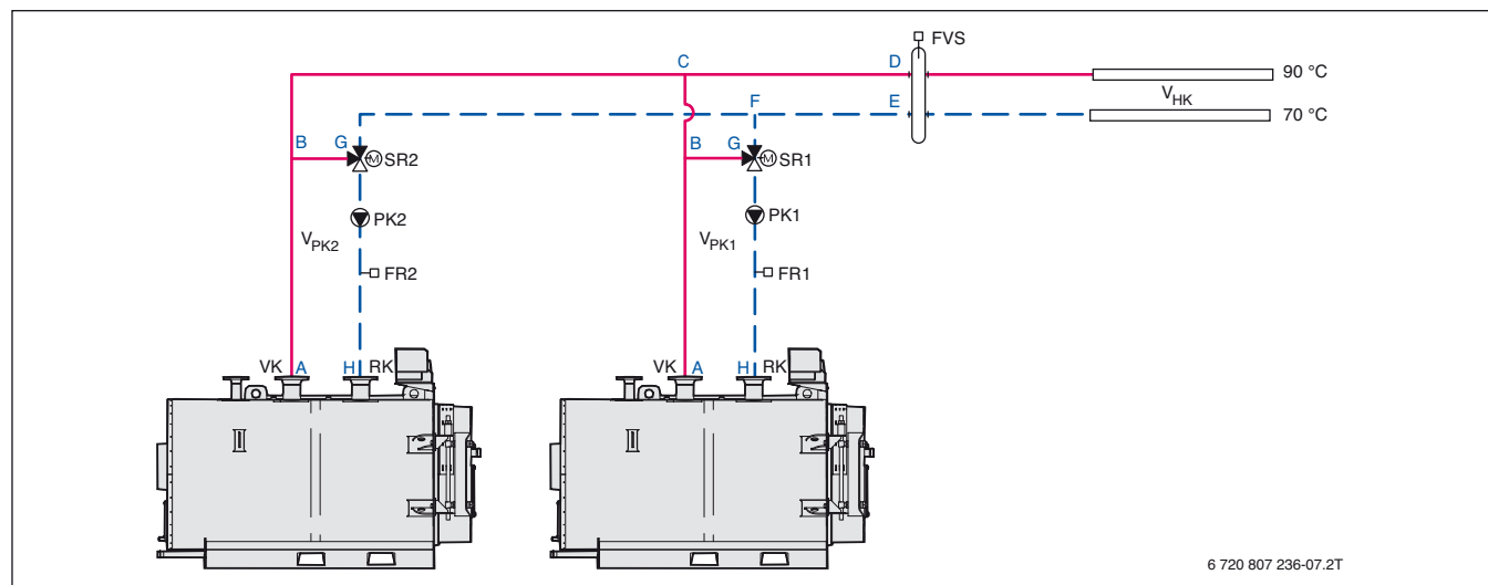
Gráfico 22 Ejemplo de circuito hidráulico para un sistema de dos calderas con bomba del circuito de caldera como bomba del circuito primario para la Uni 3000 F
