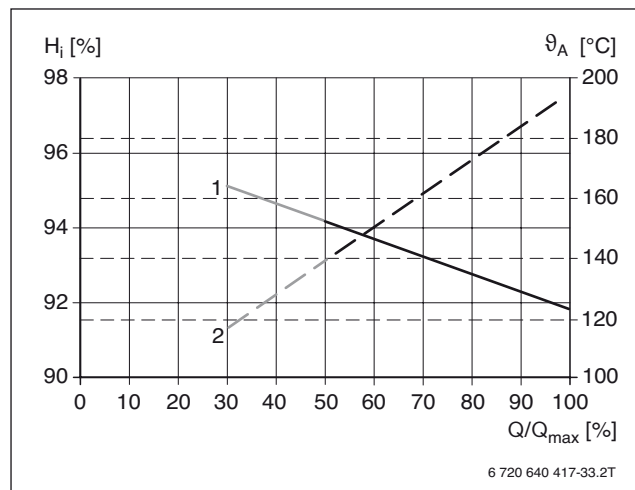
Gráfico 11 Eficiencia de la caldera y temperatura del gas de escape en relación con la carga de la caldera con una temperatura media del agua de la caldera de 70°C – Uni 3000 F
