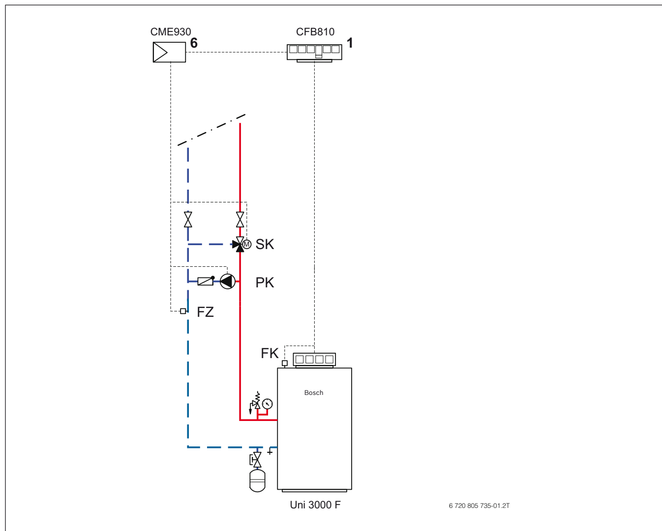
Gráfico 24 Ejemplo de sistema Uni 3000 F
