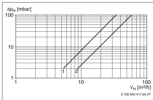
Gráfico 8 Pérdida de carga del lado del agua en la caldera Uni 3000 F
