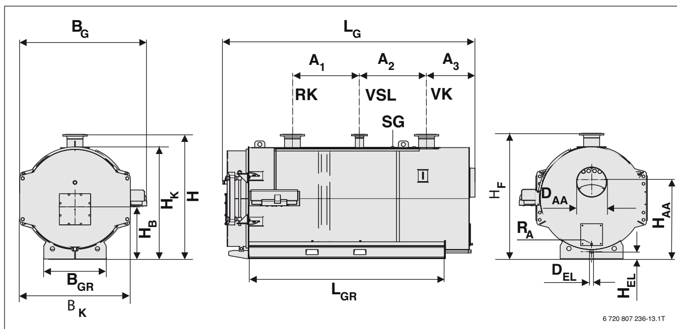
Gráfico 7 Dimensiones, Uni 3000 F 1.400 kW a 1.850 kW
