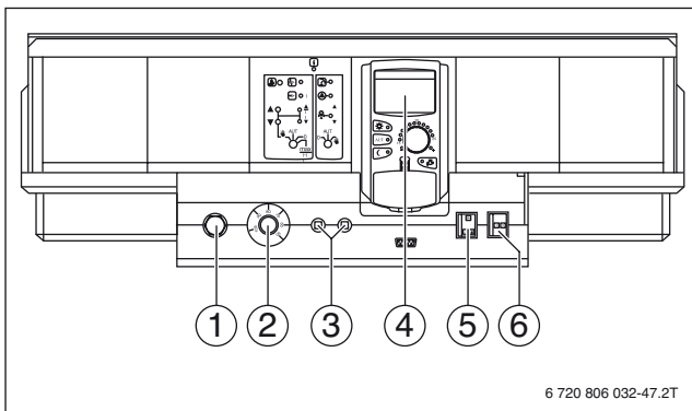
Gráfico 15 Ajustes de la unidad de regulación, ejemplo para la CFB930
