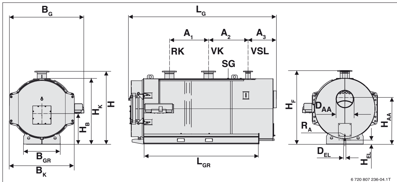
Gráfico 6 Dimensiones, Uni 3000 F 1.040 kW a 1.200 kW
