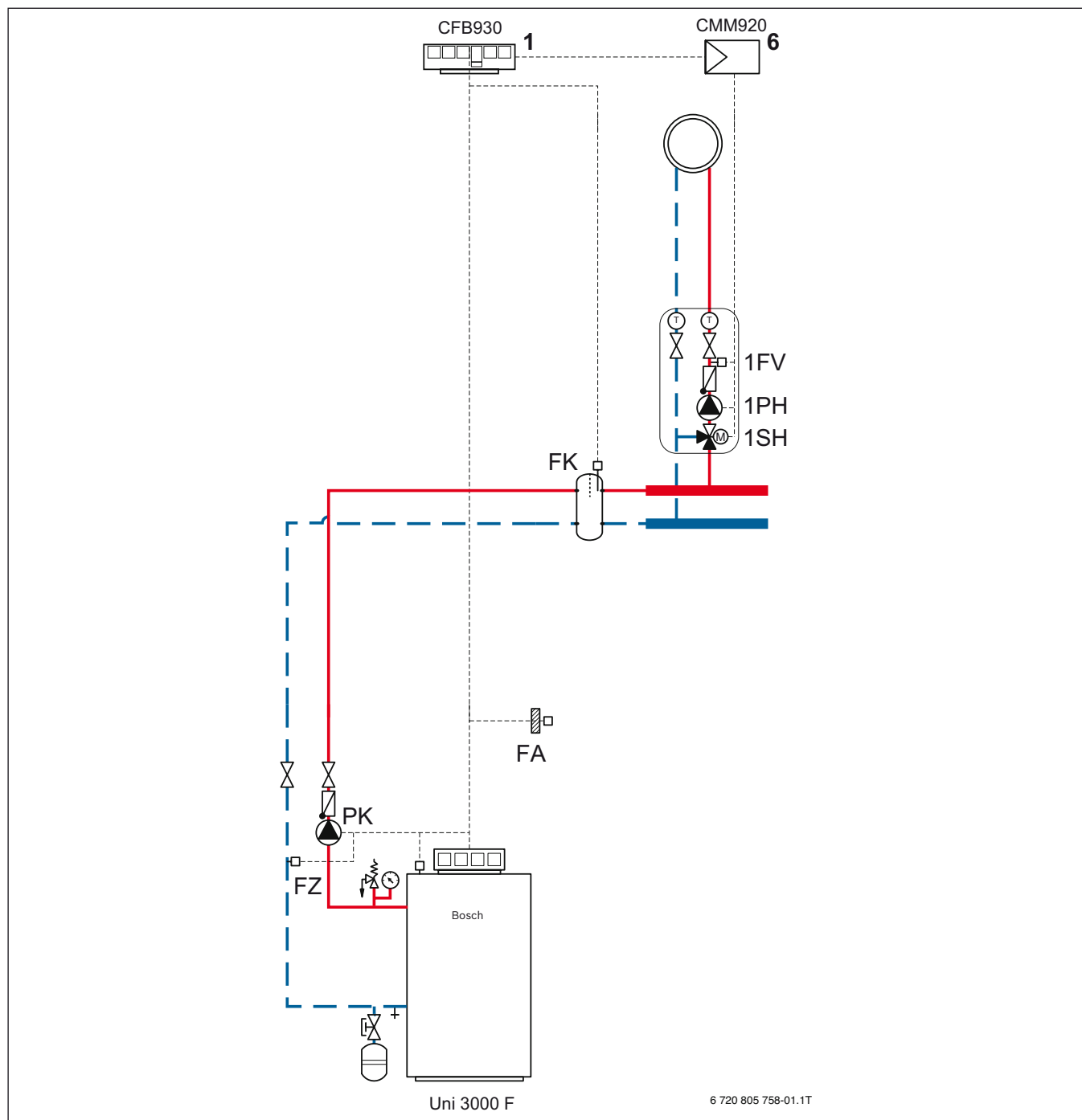
Gráfico 25 Ejemplo de sistema para Uni 3000 F con control de la caldera y del circuito de calefacción con compensador hidráulico
