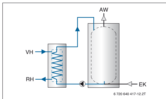
Gráfico 17 Calentamiento de A.C.S. conforme al principio de almacenamiento primario con intercambiadores externos.
