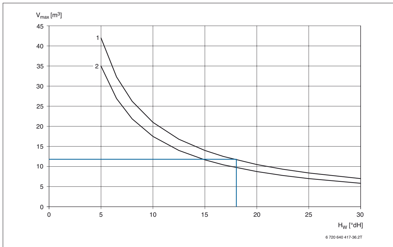
Gráfico 14 Calderas > 150 kW a 600 kW fabricadas con materiales férreos
