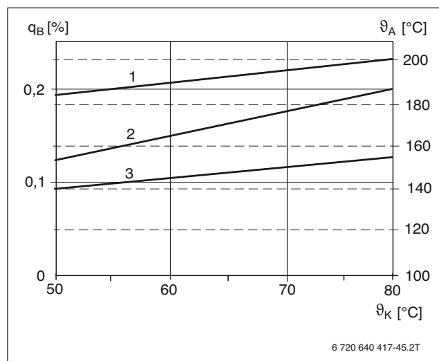
Gráfico 12 Pérdidas por disposición de servicio y temperatura del gas de escape en relación con la temperatura media del agua de la caldera - Uni 3000 F
