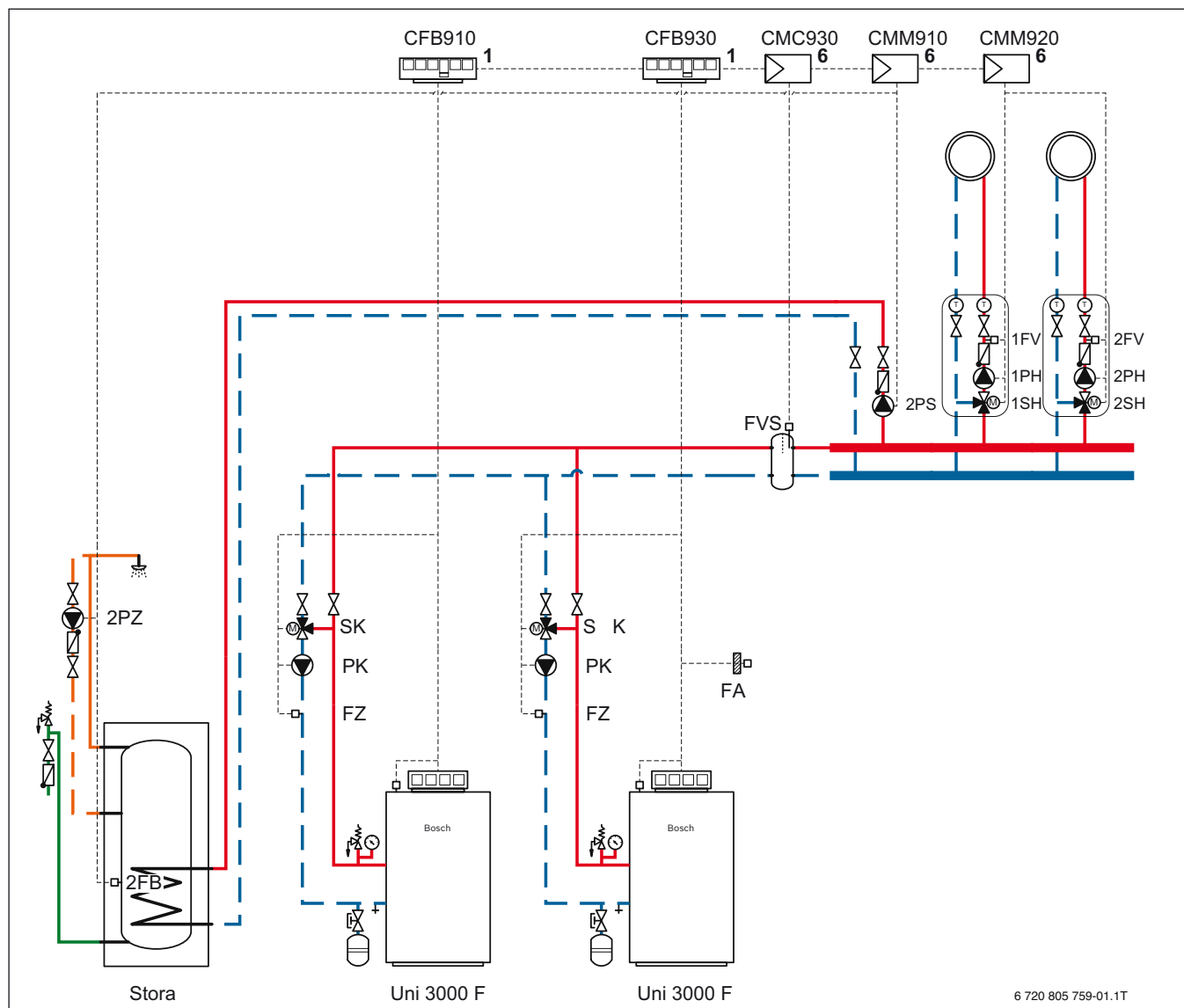
Gráfico 28 Ejemplo de sistema para Uni 3000 F
