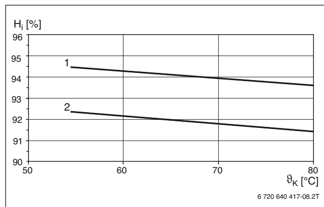
Gráfico 10 Eficiencia de la caldera en relación con la temperatura media del agua de la caldera (valor medio para todos los modelos) – Uni 3000 F
