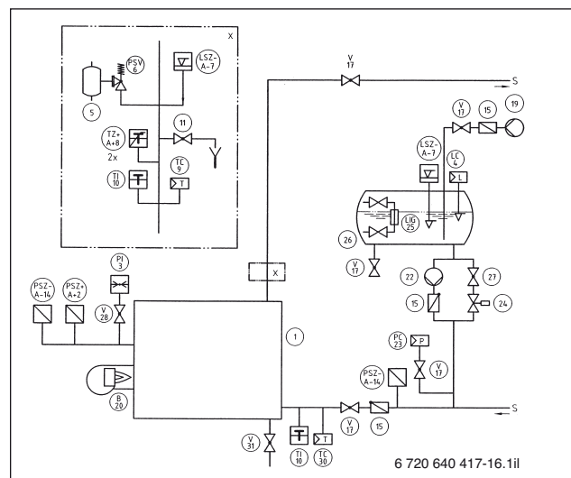
Gráfico 20 Equipamiento de seguridad conforme a la normativa EN 12953-6 para calderas con un limitador de temperatura de seguridad > 110°C; ej.: mantener la presión a través de la bomba
