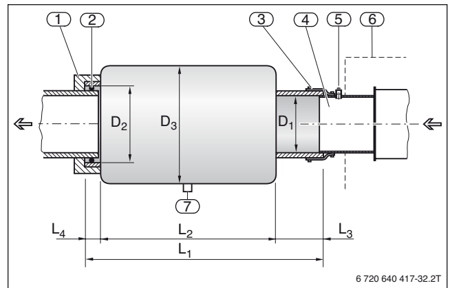
Gráfico 33 Silenciador de gases de escape con maguito de estanqueidad para el aislamiento contra ruidos
