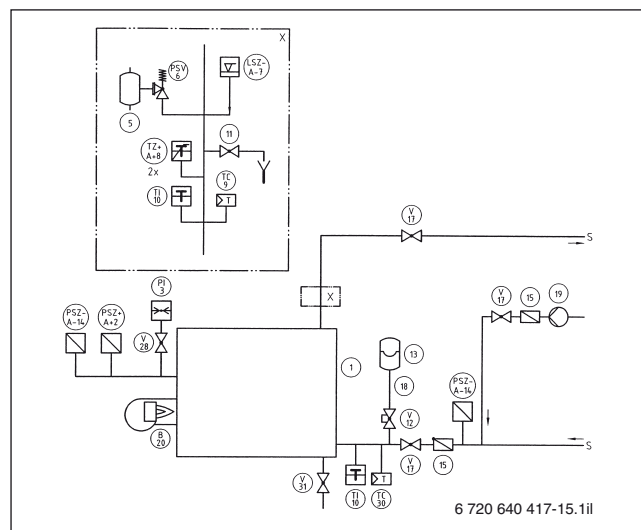
Gráfico 19 Equipamiento de seguridad conforme a la normativa EN 12953-6 para calderas con un limitador de temperatura de seguridad > 110°C; ej.: mantener la presión a través de un vaso tampón
