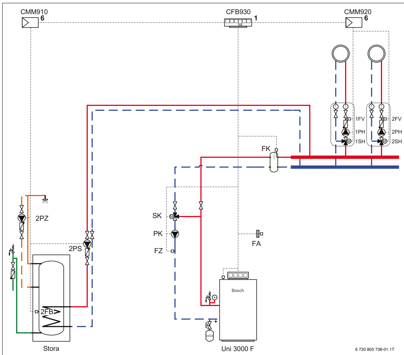
Gráfico 27 Ejemplo de sistema para Uni 3000 F
