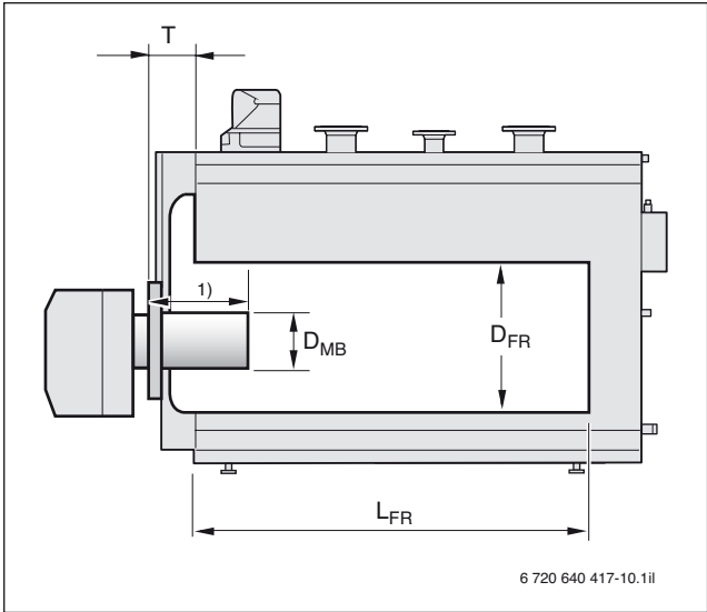
Gráfico 13 Dimensiones de instalación del quemador
