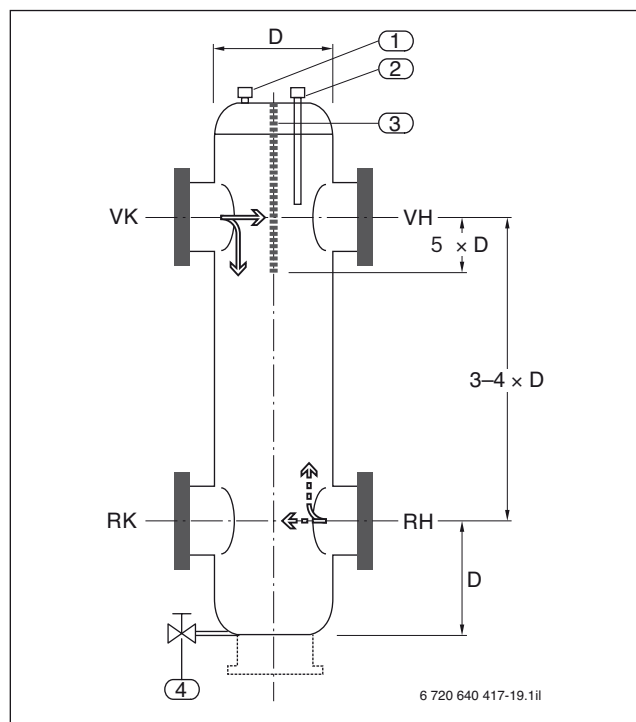
Gráfico 23 Diagrama principal de un compensador hidráulico
