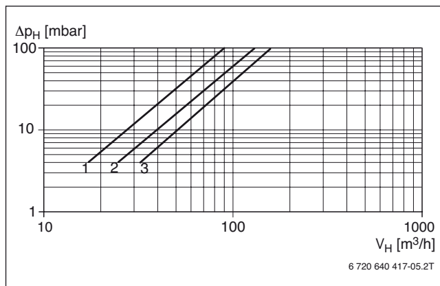
Gráfico 9 Pérdida de carga del lado del agua en la caldera Uni 3000 F
