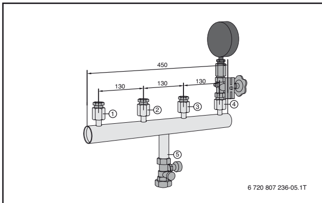
Gráfico 30 Grupo de seguridad de las calderas
