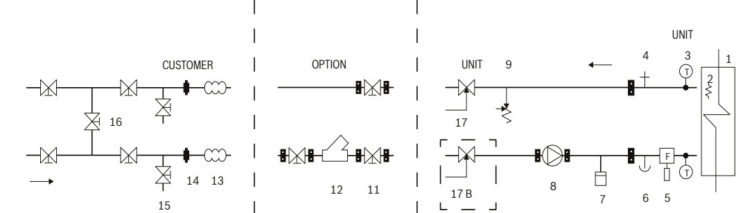
Bomba de calor con bomba de primario integrada
