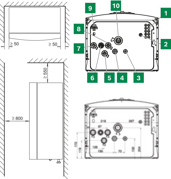
Unidad interior AWS-B (híbrida)
