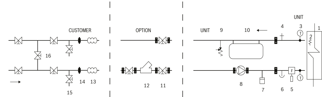
Bomba de calor con bomba de primario y depósito de inercia integrados
