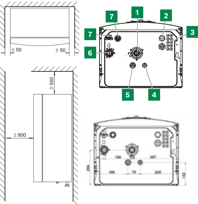
Unidad interior AWS-E (resistencia)
