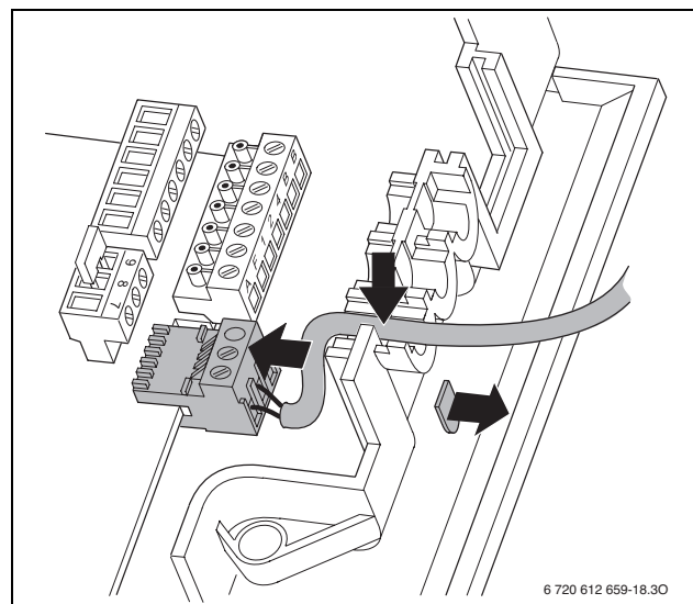
Fig. 32 Racordul senzorului pentru temperatura boilerului (NTC)
