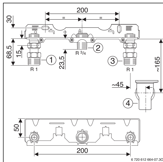
Fig. 17 Exemplu: placă de racord pentru montaj Nr. 759 la aparate ZBR
