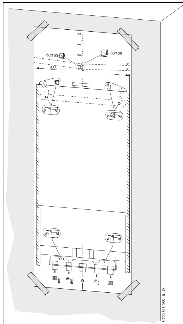
Fig. 12 Șabloane de montaj
