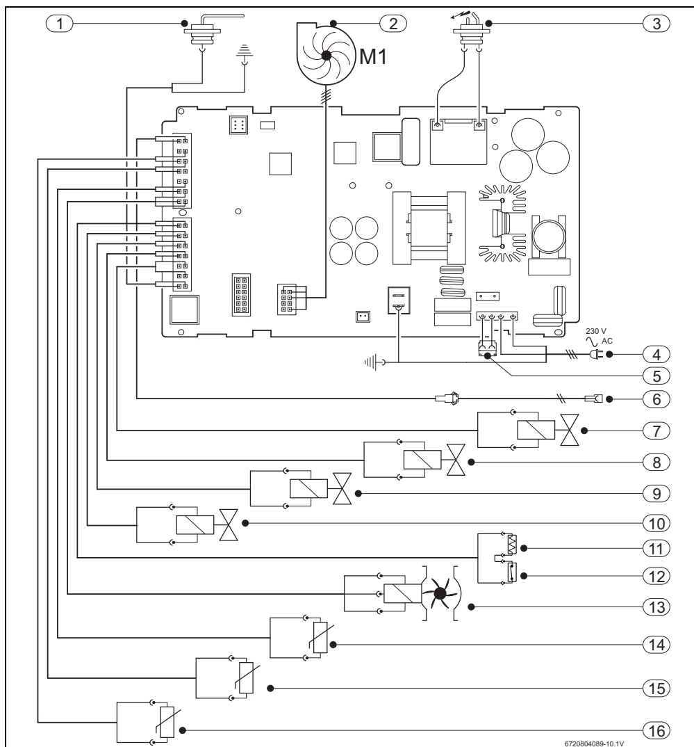
Рис. 3 Электрическая схема
