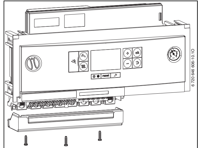
Мал. 33 Зняття кожуха
