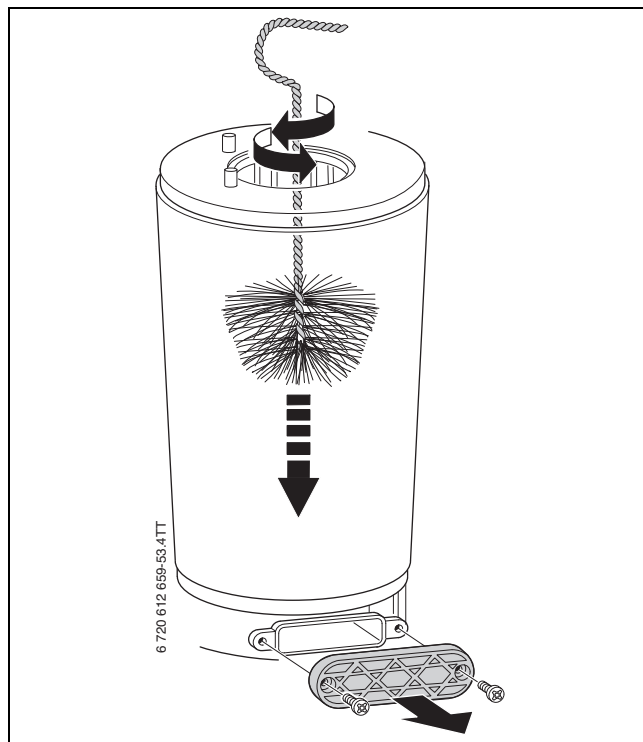
Мал. 62 Чищення теплообмінника
