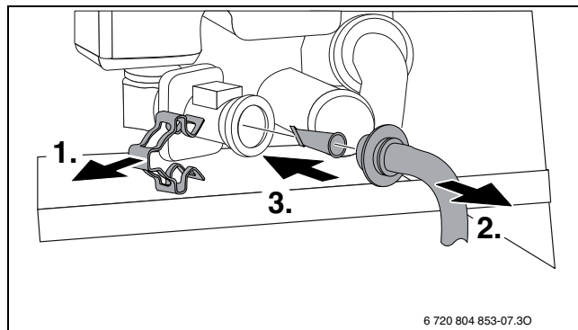
Мал. 68 Демонтаж фільтра в трубі холодної води
