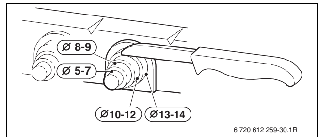
Мал. 34 Підгонка фіксатора проводу до діаметра кабелю
