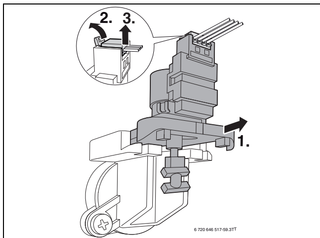
Мал. 71 Зняття мотора 3-ходового клапана
