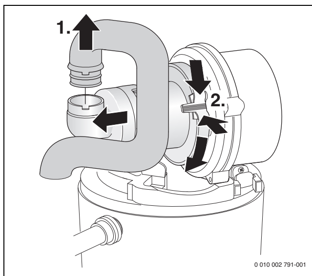
Мал. 57 Демонтаж впускної труби та змішувальної камери
