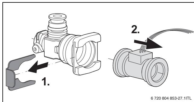
Мал. 69 Демонтаж турбіни на трубі холодної води
