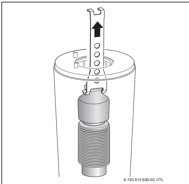
Мал. 60 Виймання верхнього елемента теплообмінника, що служить для оптимізації розподілювання тепла
