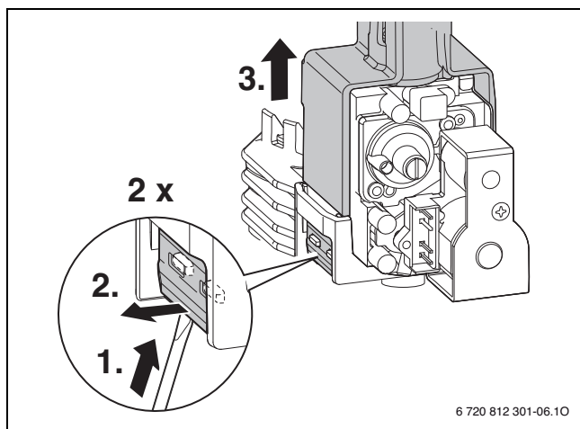
Мал. 75 Демонтаж газової арматури
