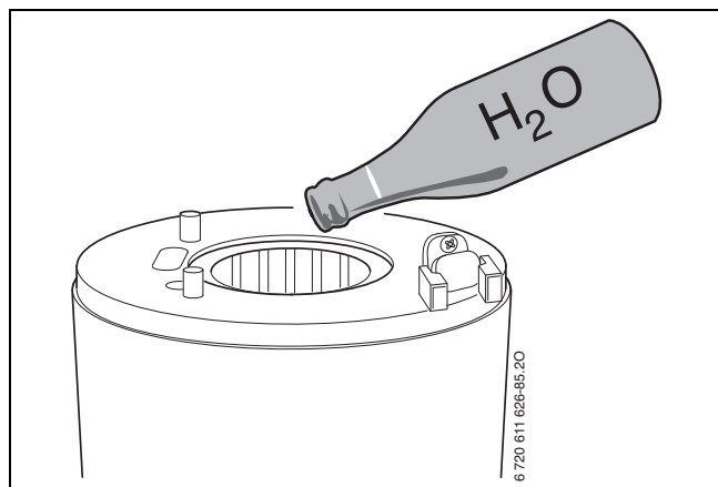
Мал. 64 Промивання водою котлового блока, який включає камеру згорання і теплообмінник
