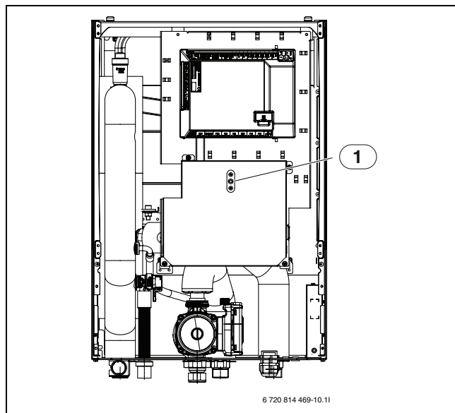
Rys. 7 Jednostka wewnętrzna AWES
