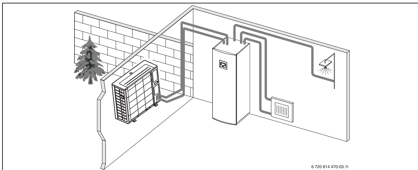
Rys. 1 Pompa ciepła (jednostka zewnętrzna), jednostka wewnętrzna AWMS/AWMSS ze zintegrowanym podgrzewaczem pojemnościowym c.w.u. i dogrzewaczem elektrycznym
