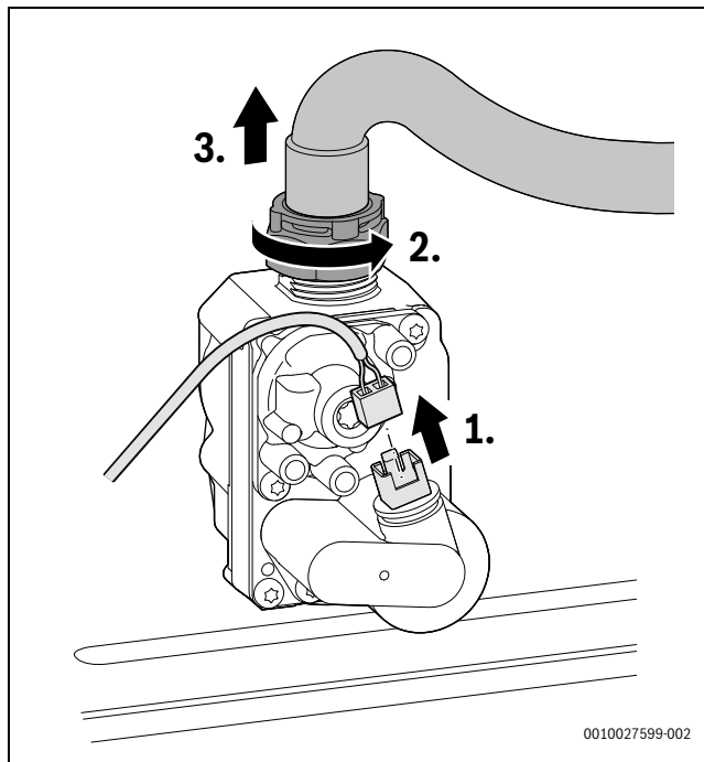
Fig. 71 Scollegamento del connettore dalla valvola del gas e rimozione del dado a risvolto con il tubo flessibile del gas
