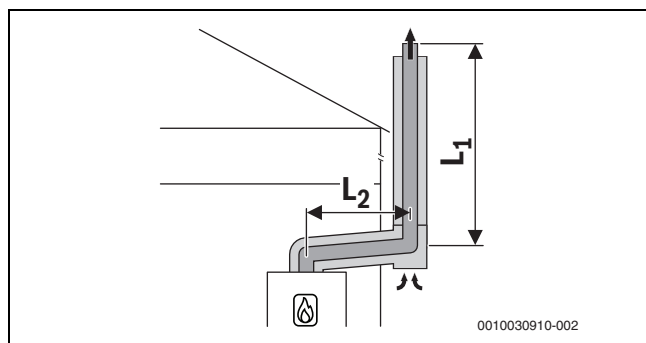
Fig. 14 Condotta di aspirazione aria comburente/evacuazione prodotti della combustione concentrico secondo C_{53x} sulla parete esterna
