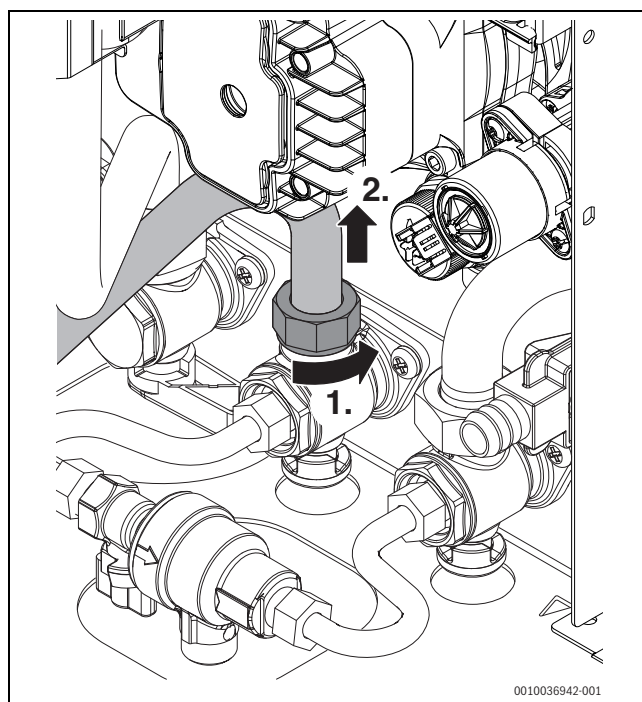
Fig. 69 Togliere il tubo sul raccordo acqua fredda sanitaria
