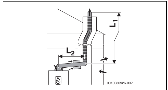
Fig. 18 Condotto combusti intubato in cavedio, flessibile, secondo B_{23p}/B_{53p} con adduzione aria comburente sull'apparecchio dipendente dall'aria del locale ed elemento di collegamento concentrico tra luogo di posa e cavedio
