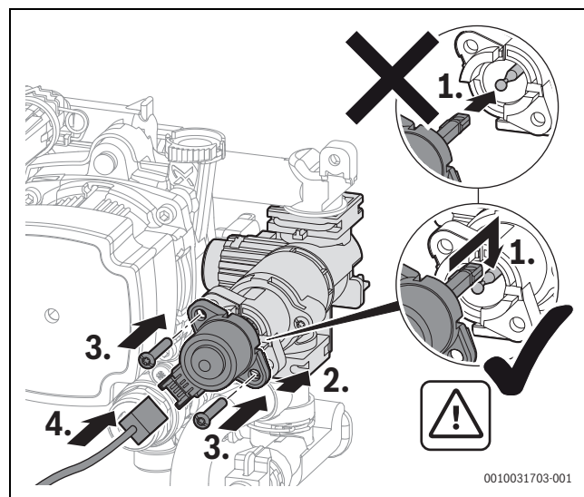
Fig. 82 Montare il motore sulla valvola a 3 vie (variante con viti)
