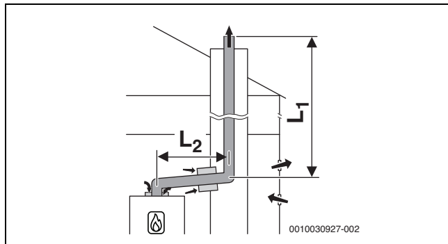
Fig. 17 Condotto combusti intubato in cavedio, rigido, secondo B_{23p}/B_{53p} con adduzione aria comburente sull'apparecchio dipendente dall'aria del locale ed elemento di collegamento concentrico tra luogo di posa e cavedio
