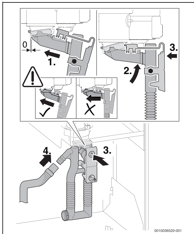
Fig. 68 Applicazione del sifone per la condensa
