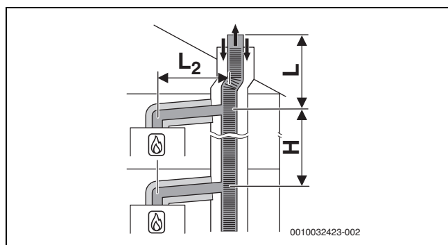
Fig. 22 Collettore scarico combusto secondo C_{(14)3x} con condotto di evacuazione prodotti della combustione collettivo e condotto di aspirazione aria comburente/evacuazione prodotti della combustione concentrico nel luogo di posa
