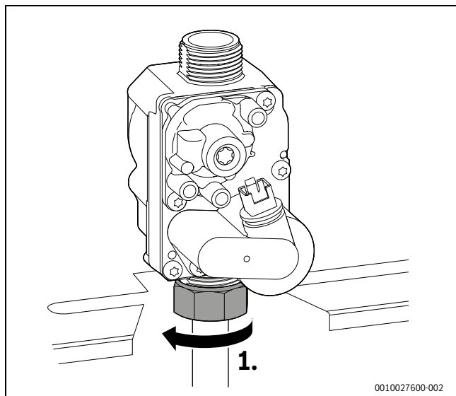
Fig. 73 Svitamento del dado a risvolto
