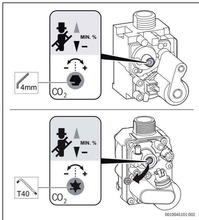
Fig. 47 Taratura del tenore di \text{CO}_2/\text{O}_2 a potenza termica nominale minima
