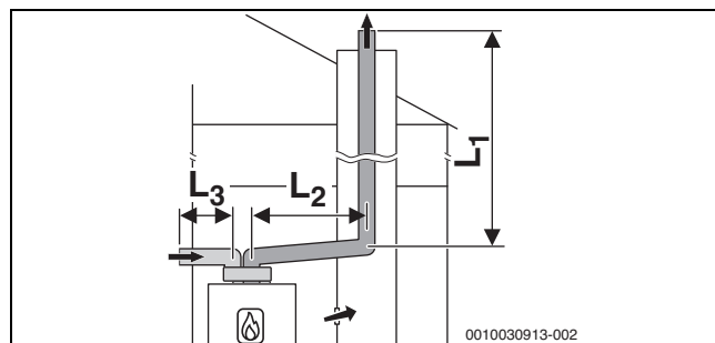
Fig. 12 Sistema di aspirazione aria/evacuazione pdc rigido secondo C 53 nel cavedio e condotto di aspirazione aria comburente/evacuazione pdc con tubi separati per adduzione aria ed evacuazione pdc nel luogo di posa
