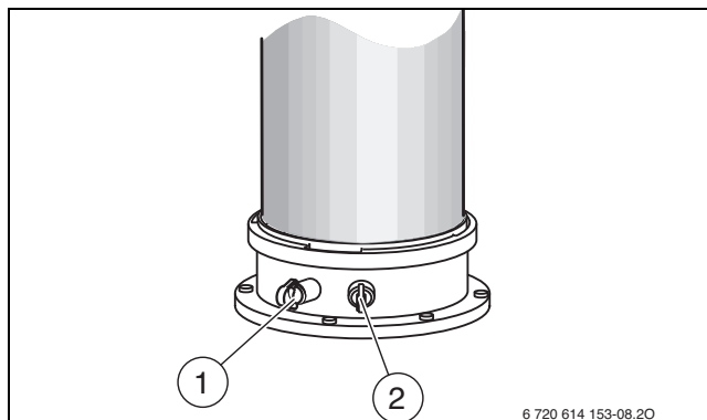
Fig. 48 Tronchetto di misurazione gas combustibili e tronchetto di misurazione per aria comburente
