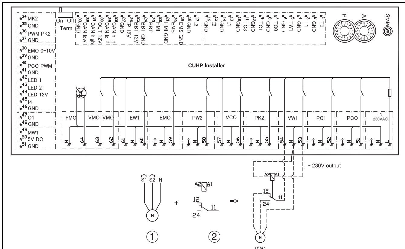
Joon. 38 Kolmesuunalise ümberlülitatava klapi alternatiivne paigaldamine
