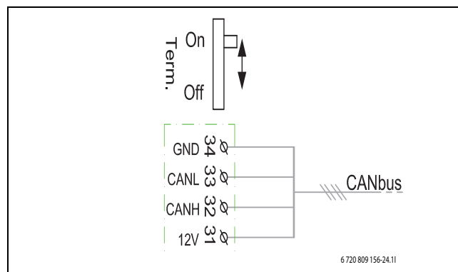
Joon. 9 CAN-BUS-i termineerimine (lõpptakistiga varustamine)
