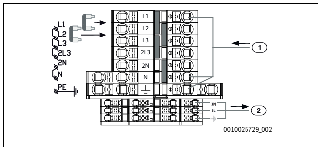
Joon. 13 Alternatiivversioon
