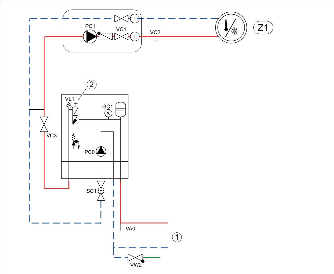
Joon. 21 Integreeritud elektrilise lisakütteseadme ja küttesüsteemiga siseüksus
