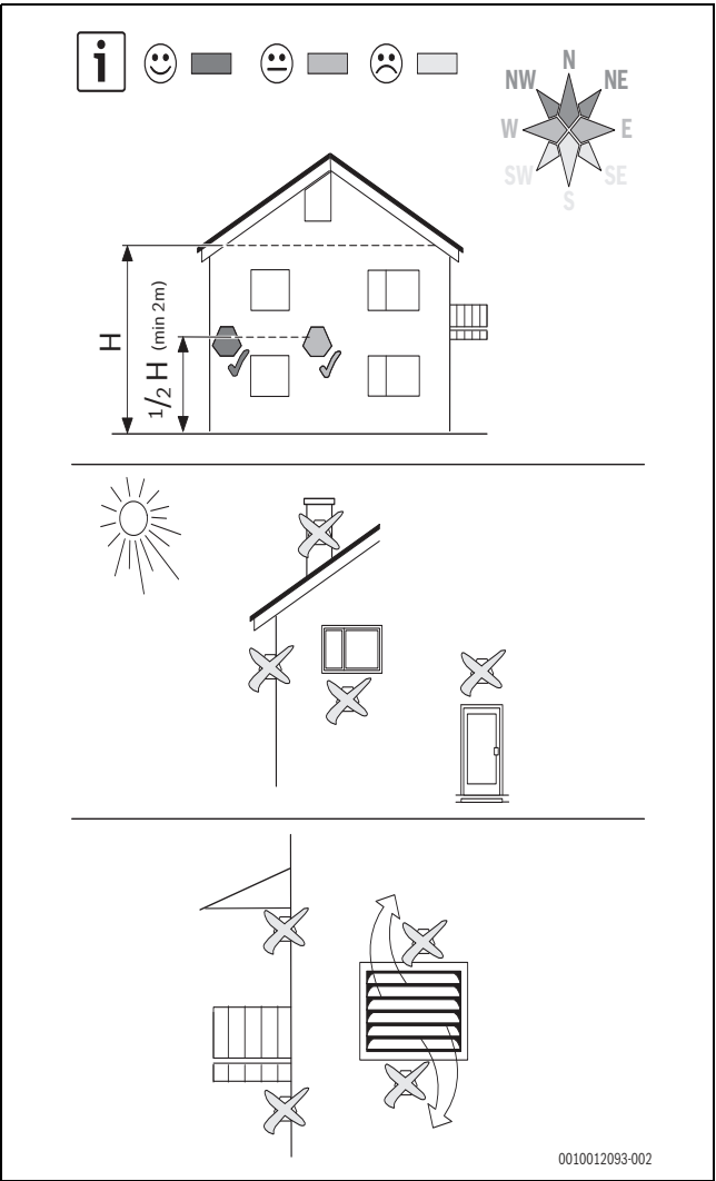
Joon. 10 Välitemperatuuri anduri paigaldus
