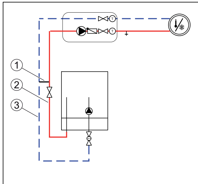
Joon. 31 Siseüksus koos küttekontuuri ja mõõdaviiguga
