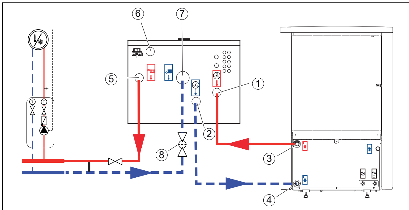
Joon. 7 Elektrilise lisakütte süsteemiga siseüksuse ühendamine soojuspumba ja küttesüsteemiga
