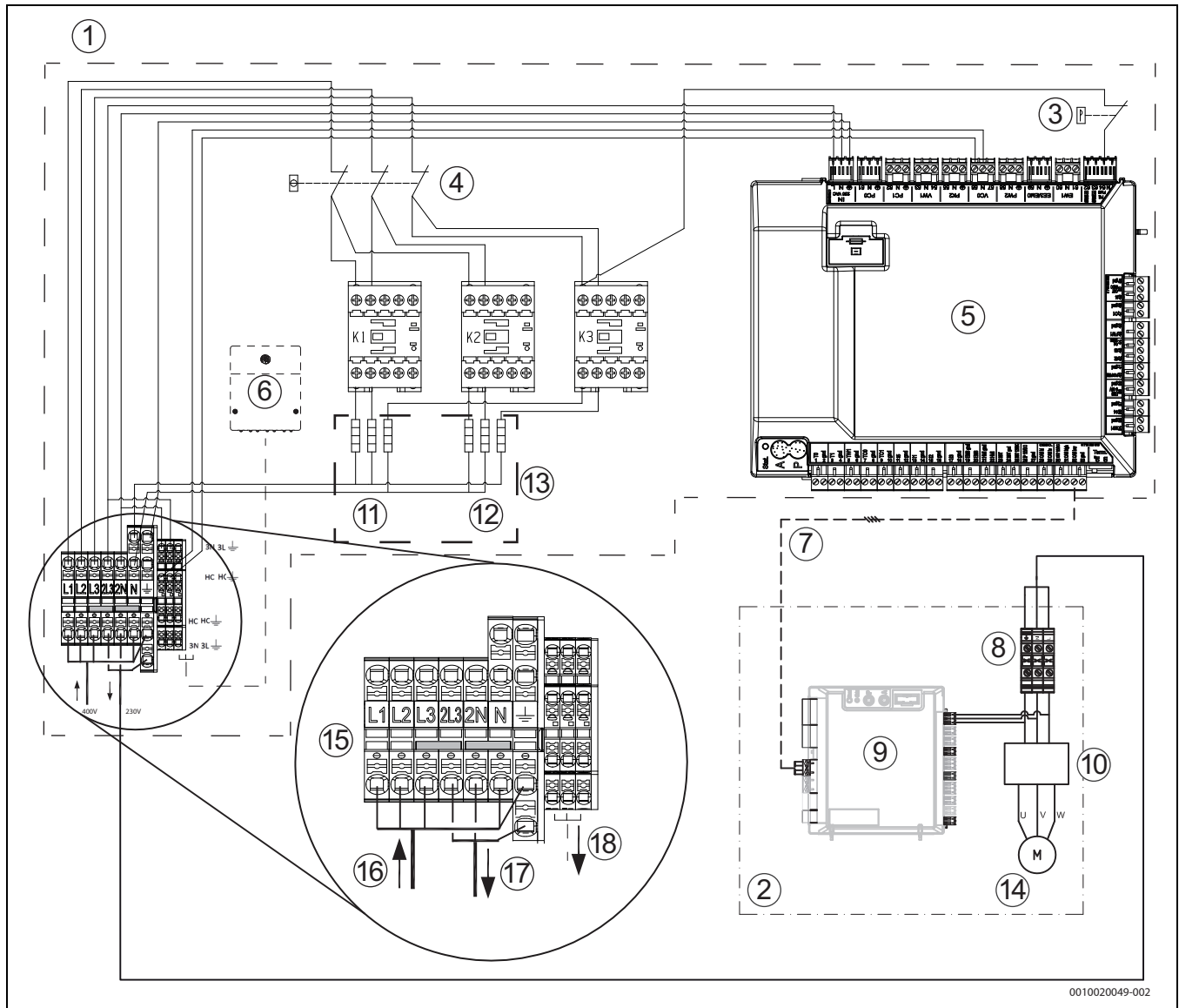
Joon. 35 Integreeritud elektrilise lisaküttesüsteemiga (kolmefaasiline vool) ühefaasiline soojuspump
