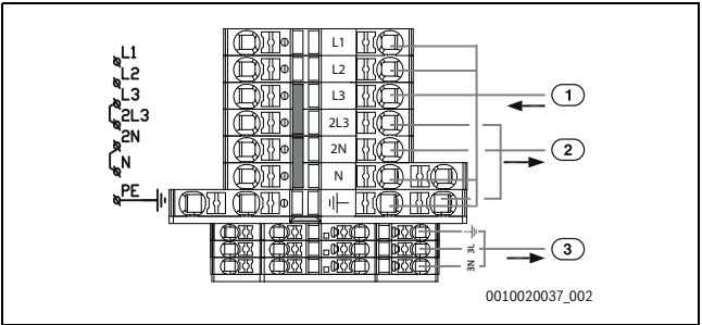
Joon. 12 Standardne elektriühendus integreeritud elektrilise lisaküttesüsteemi korral
