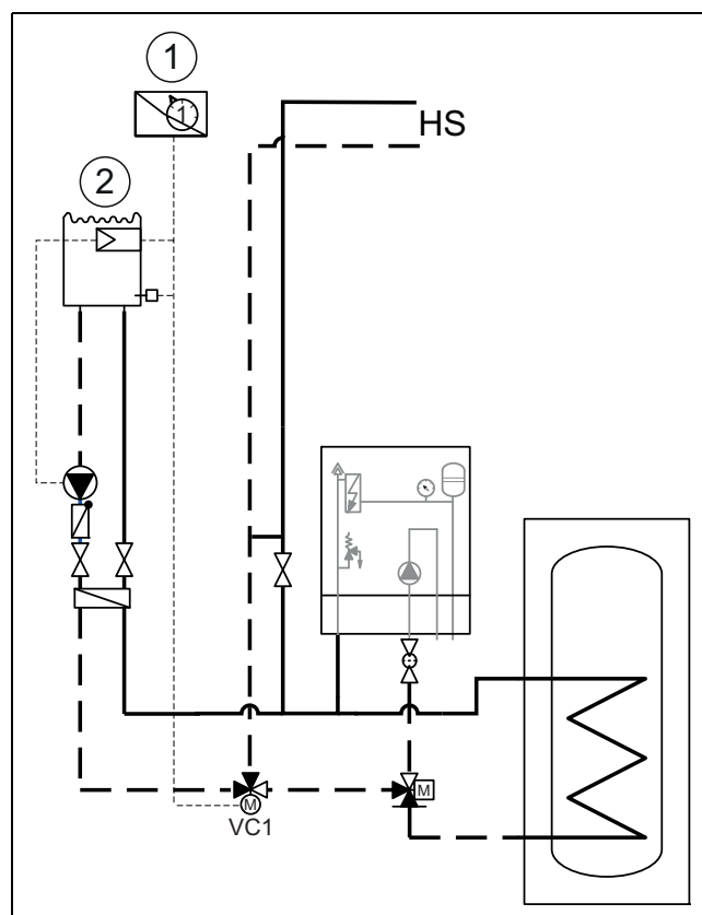
Joon. 29 Basseini paigaldamise näidisjoonis
