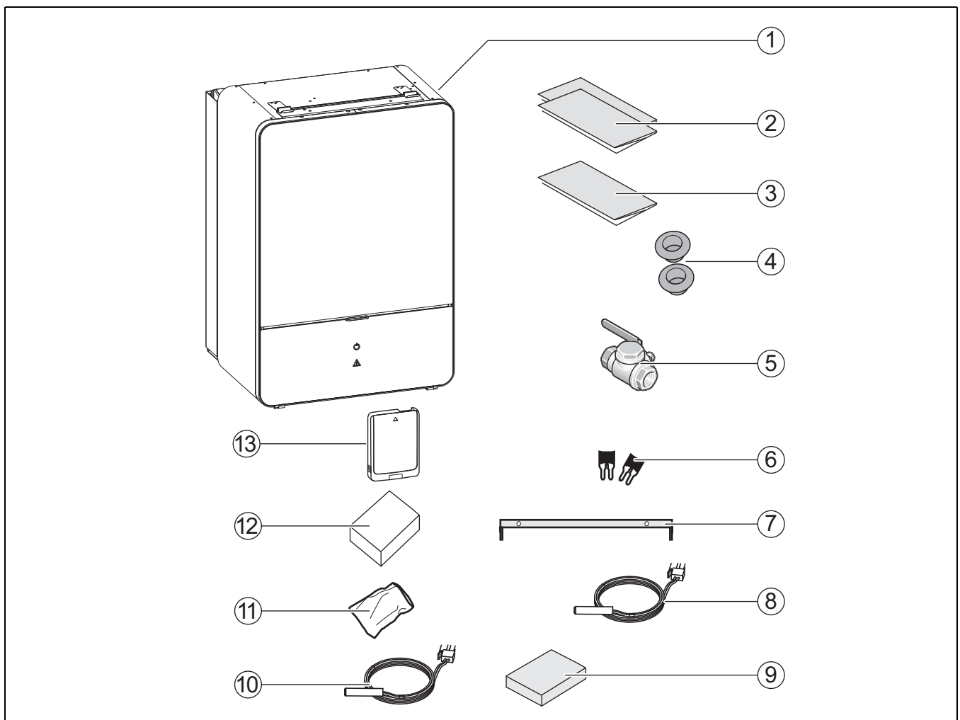
Joon. 2 Tarnekomplekt
