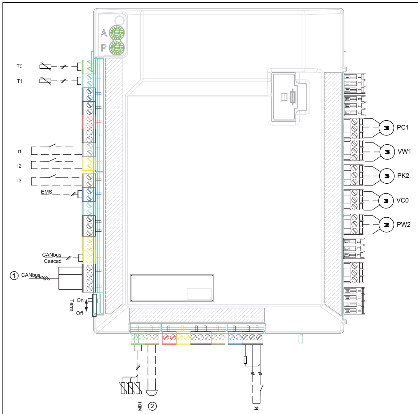
Joon. 14 Paigaldusmooduli ühendused
