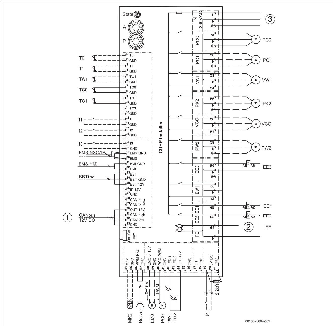
Joon. 37 Integreeritud elektrilise lisaküttesüsteemiga paigaldusmooduli ühendusskeem
