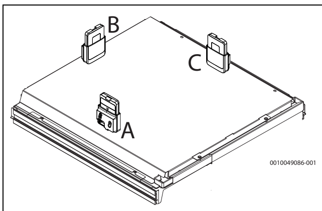
Joon. 17 Ühendusdetaili kinnitamine siseüksuse ülaosale. Lisaks ühendusdetailile on joonisel kujutatud ka Radiomoodul, mis asub ühendusdetaili sees
