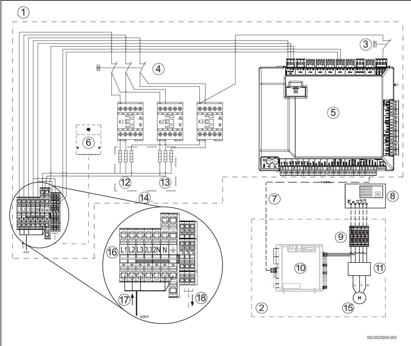
Joon. 36 Integreeritud elektrilise lisaküttesüsteemiga (kolmefaasiline vool) soojuspump (kolmefaasiline vool)
