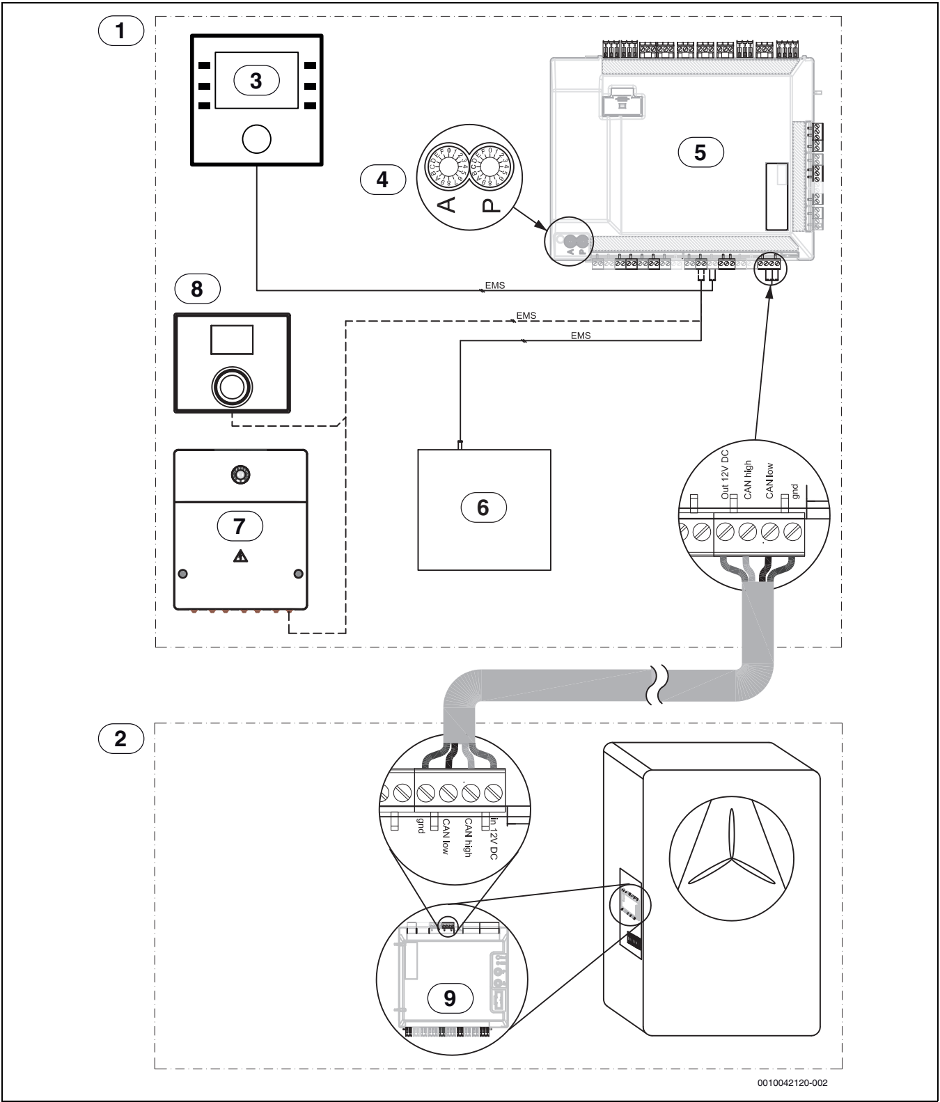
Joon. 34 CAN-BUS/EMS-BUS siseüksusele koos elektrilise lisaküttesüsteemiga - ülevaade
