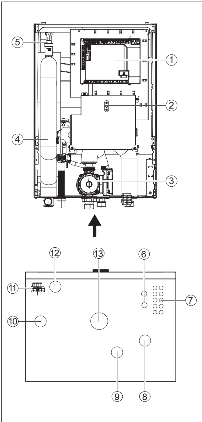
Joon. 3 Lisakütteseadmega siseüksuse osad ja toruühendused
