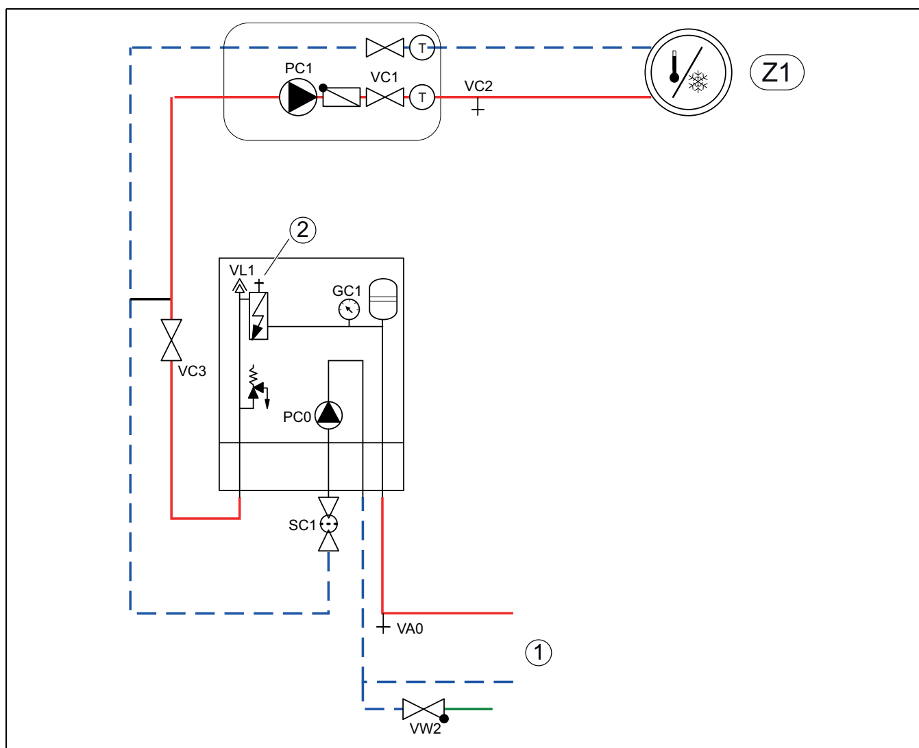
Joon. 8 Integreeritud elektrilise lisakütteseadme ja küttesüsteemiga siseüksus
