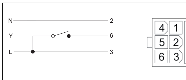
Joon. 28 Molex-pistik
