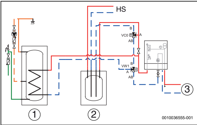
Joon. 30 Puhver, VCO-möödaviiguventiil
