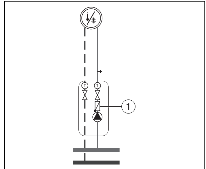
Joon. 32 Küttekontuur
