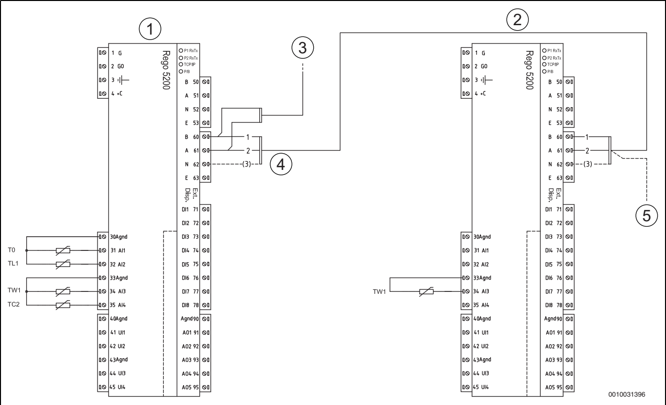
Fig. 33 El-diagram, serieforbundet
