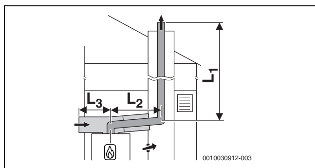
Rys. 28 Sztywne odprowadzenie spalin wg C 53x w szachcie i instalacja powietrzno-spalinowa z oddzielnym doprowadzeniem powietrza i koncentrycznym odprowadzeniem spalin w pomieszczeniu zainstalowania
