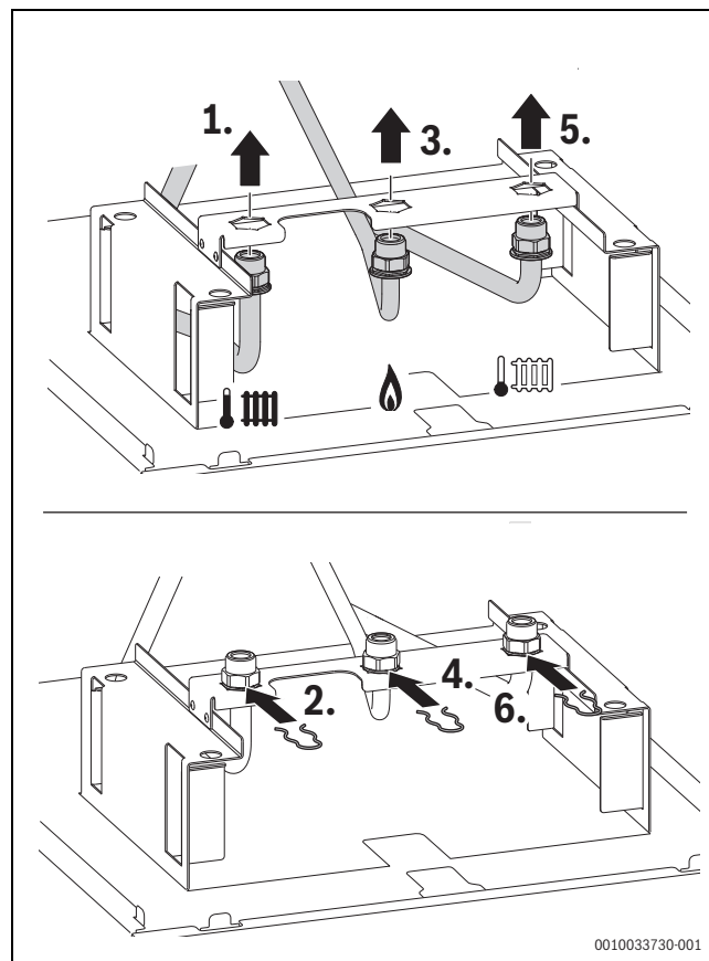
Rys. 56 Podłączanie zasilania instalacji grzewczej, rury gazowej i powrotu instalacji grzewczej z przodu (osprzęt dodatkowy CS 35)
