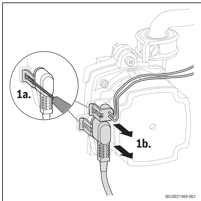
Rys. 141 Odłączanie wtyczki od pompy c.o.
