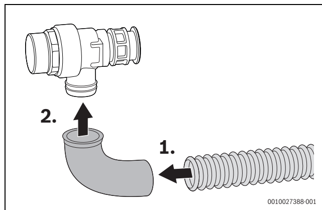
Rys. 75 Podłączanie węża do zaworu bezpieczeństwa
