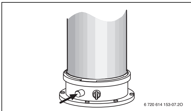
Rys. 112 Zdejmowanie korka
