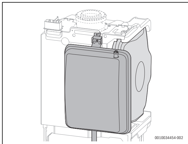
Rys. 47 2 naczynia wzbiorcze zamontowane w urządzeniu
