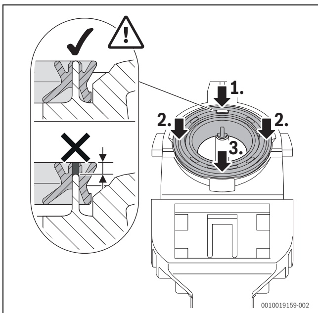
Rys. 156 Dociśnięcie uszczelki
