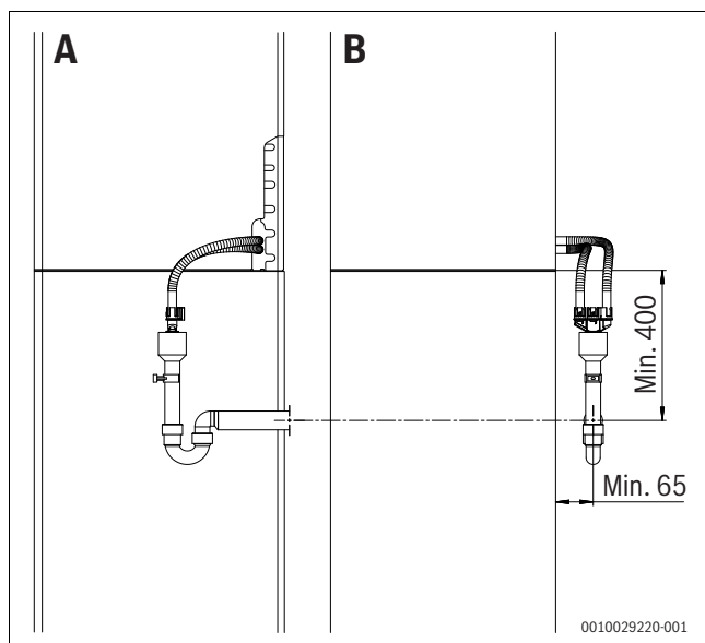
Rys. 19 A: Widok z prawej strony (wymiary w mm) B: Widok z przodu (wymiary w mm)
