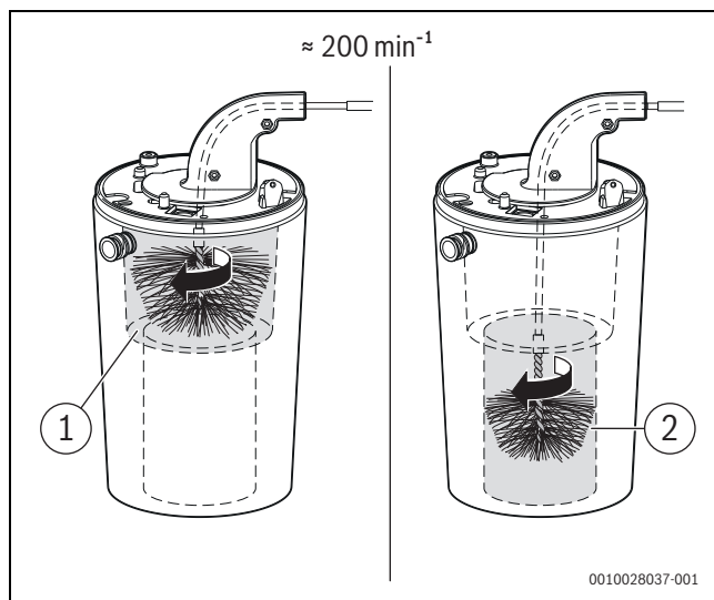
Rys. 135 Czyszczenie bloku ciepłego (ok. 200 min -1 , tylko ruch w prawo)
