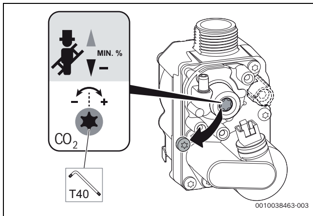
Rys. 114 Ustawianie stężenia \text{CO}_2/\text{O}_2 dla minimalnej znamionowej mocy cieplnej
