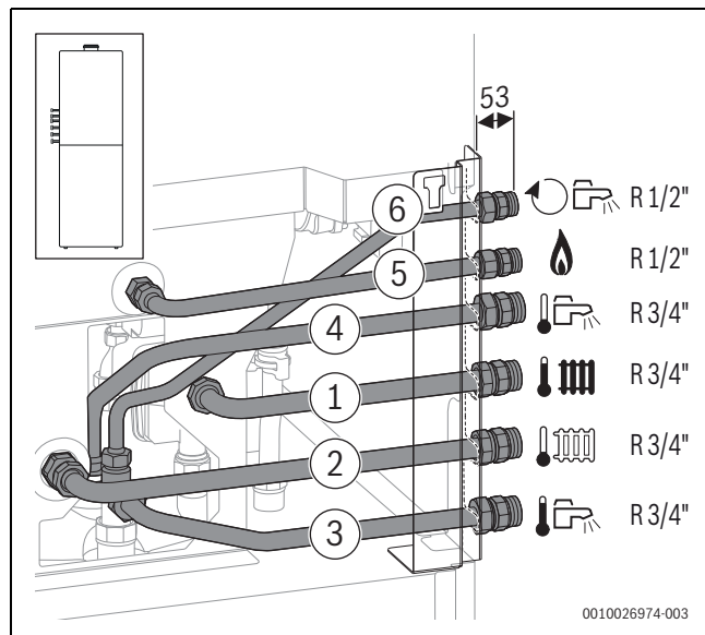
Rys. 58 Osprzęt dodatkowy CS 10 zamontowany z lewej strony
