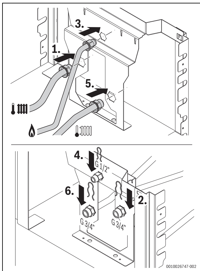
Rys. 55 Podłączanie zasilania instalacji grzewczej, rury gazowej i powrotu instalacji grzewczej z tyłu (osprzęt dodatkowy CS 35)
