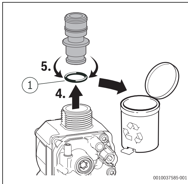
Rys. 146 Zdejmowanie dyszy gazowej
