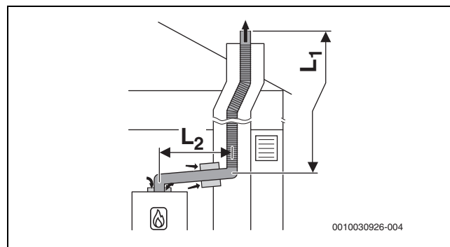
Rys. 37 Elastyczne prowadzenie spalin w szachcie zgodnie z B 53p z dopływem powietrza zależnym od powietrza w pomieszczeniu przy urządzeniu i koncentrycznej złączce między pomieszczeniem instalacyjnym a szachtem
