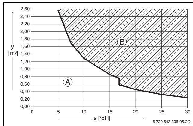
Rys. 44 Wymagania dotyczące wody do napełniania i uzupełniania w °dH do urządzeń o mocy < 50 kW
