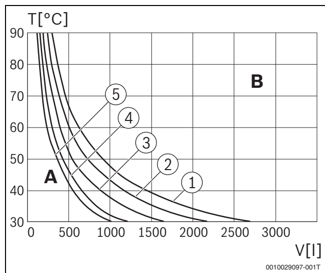
Rys. 48 Krzywe charakterystyki naczynia wzbiorczego (29 l)
