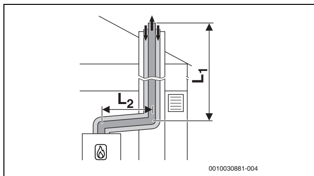
Rys. 25 Koncentryczna instalacja powietrzno-spalinowa wg C 33x w szachcie
