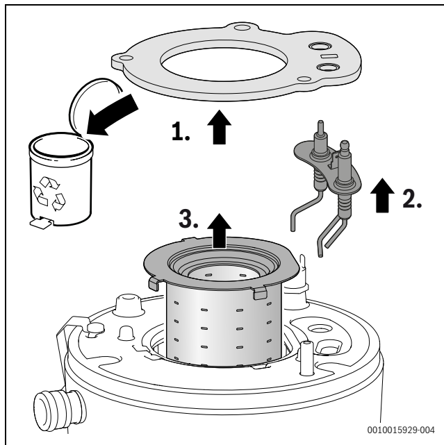
Rys. 130 Wyjmowanie palnika
