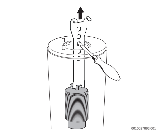
Rys. 132 Wyjmowanie dolnego elementu wyporowego
