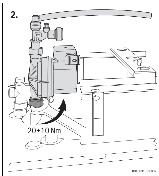
Rys. 52 Przestrzeganie momentu dokręcenia
