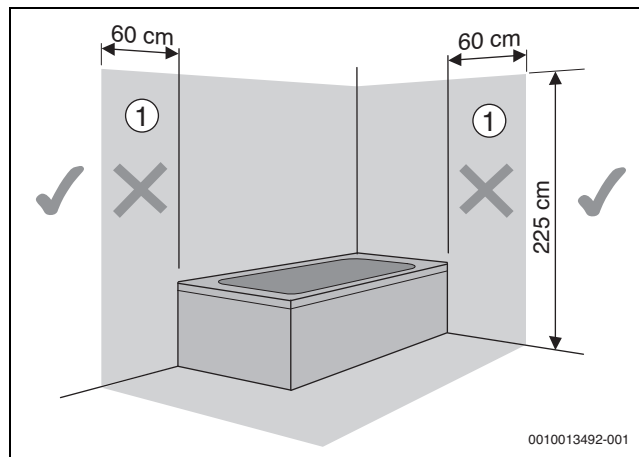
Rys. 43 Strefy ochronne
