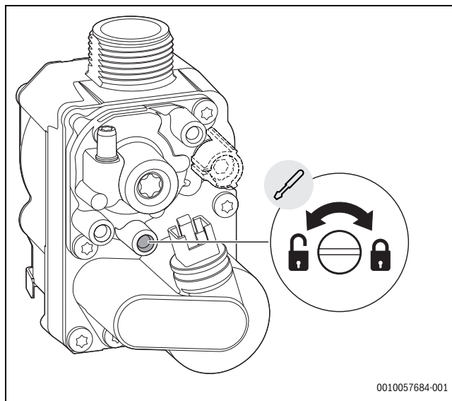
Rys. 111 Pomiar ciśnienia gazu na przyłączy
