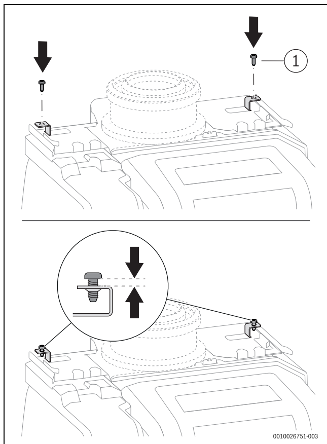
Rys. 61 Luźne wkręcanie śrub w górnej części obudowy
