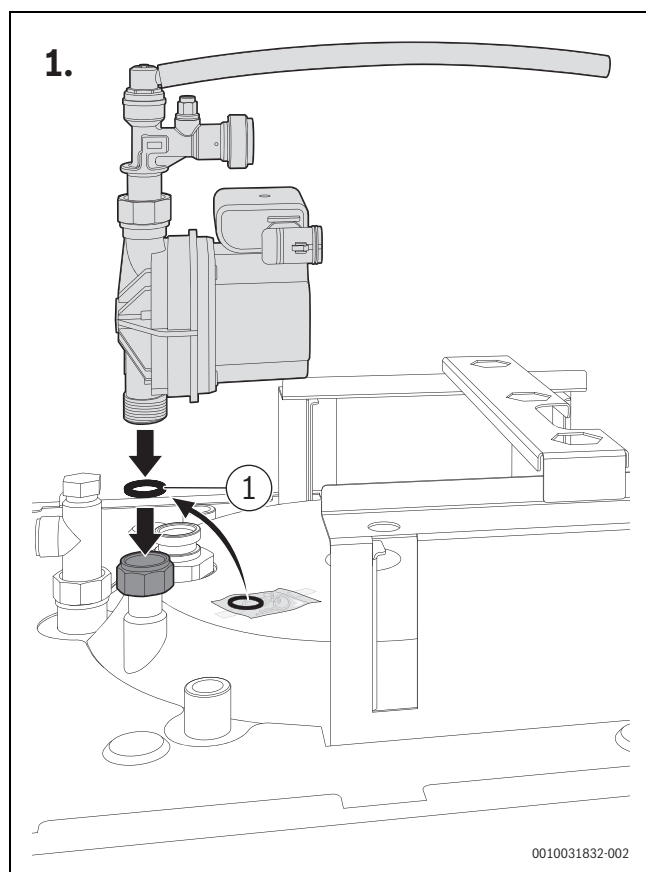
Rys. 51 Wkładanie pompy ładującej warstwowo
