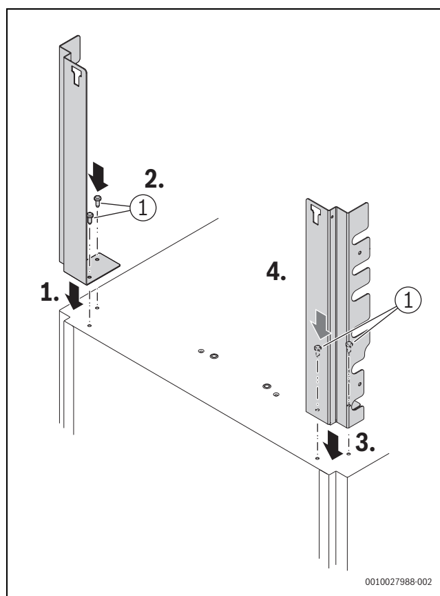
Rys. 53 Montaż Modułu bazowego (osprzęt dodatkowy CS 35) – krok 1
