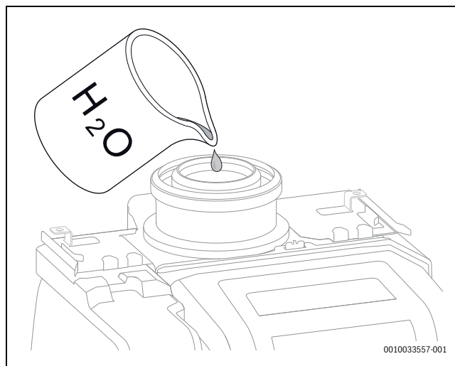
Rys. 78 Napełnianie syfonu kondensatu wodą
