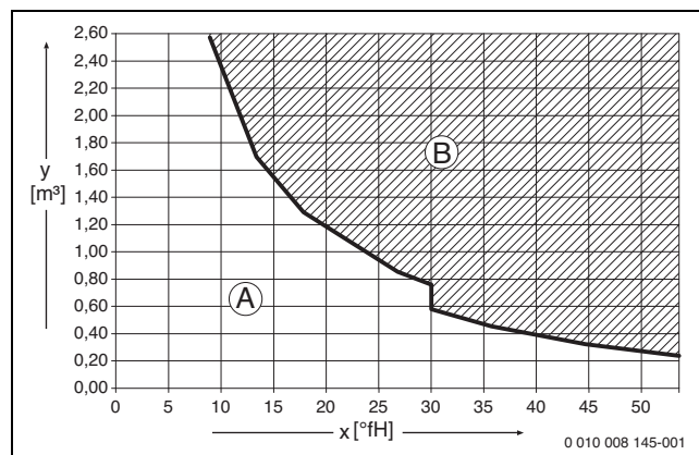
Rys. 45 Wymagania dotyczące wody do napełniania i uzupełniania w °fH do urządzeń o mocy < 50 kW
