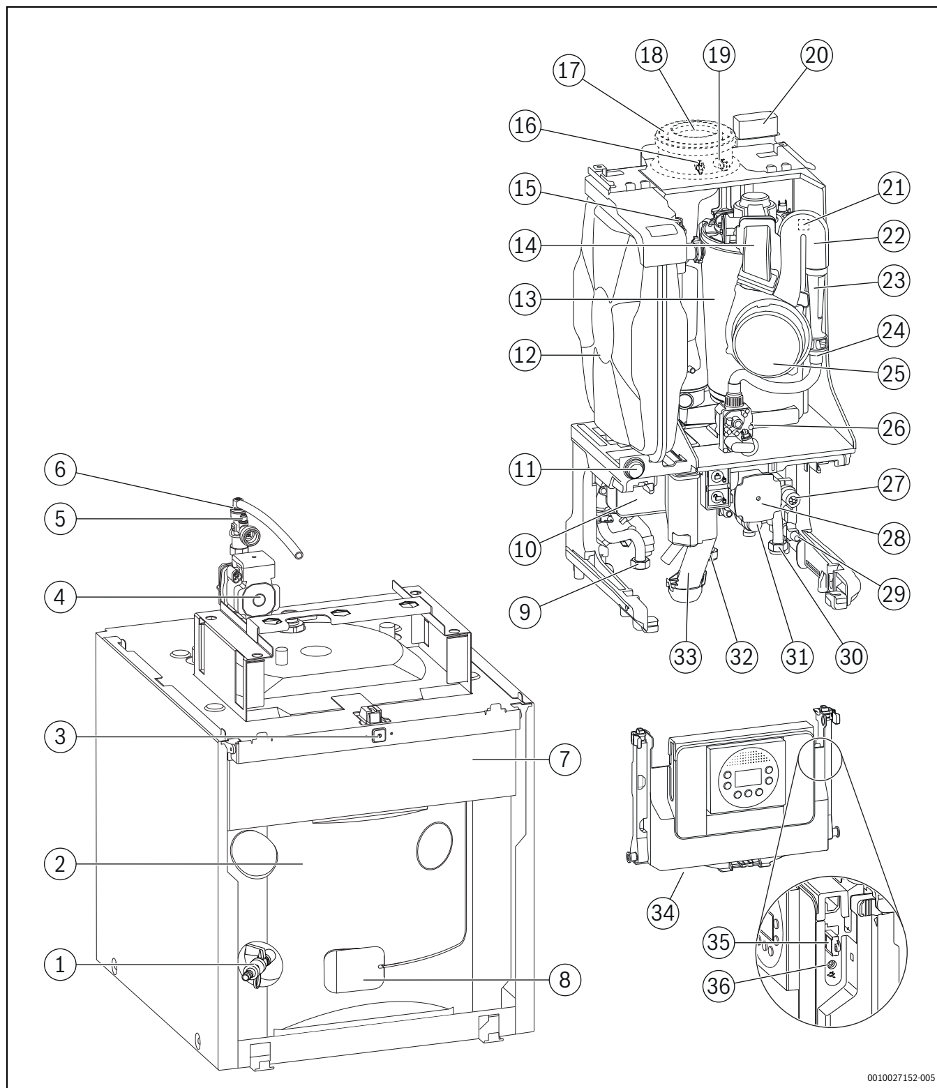
Rys. 5 Przegląd produktu
