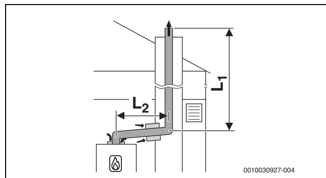
Rys. 35 Sztywne prowadzenie spalin w szachcie zgodnie z B 53p z dopływem powietrza zależnym od powietrza w pomieszczeniu przy urządzeniu i koncentrycznej złączce między pomieszczeniem instalacyjnym a szachtem
