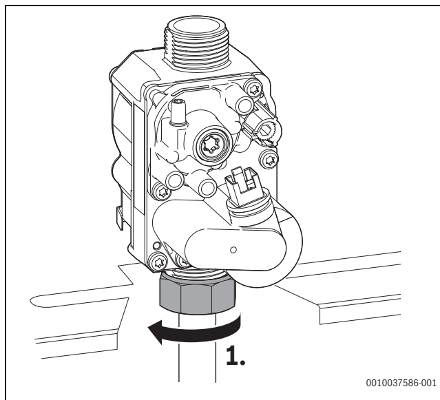
Rys. 147 Luzowanie nakrętki złączkowej
