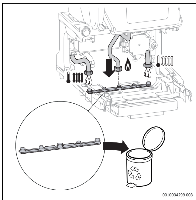
Rys. 62 Demontaż listwy osłonowej z urządzenia
