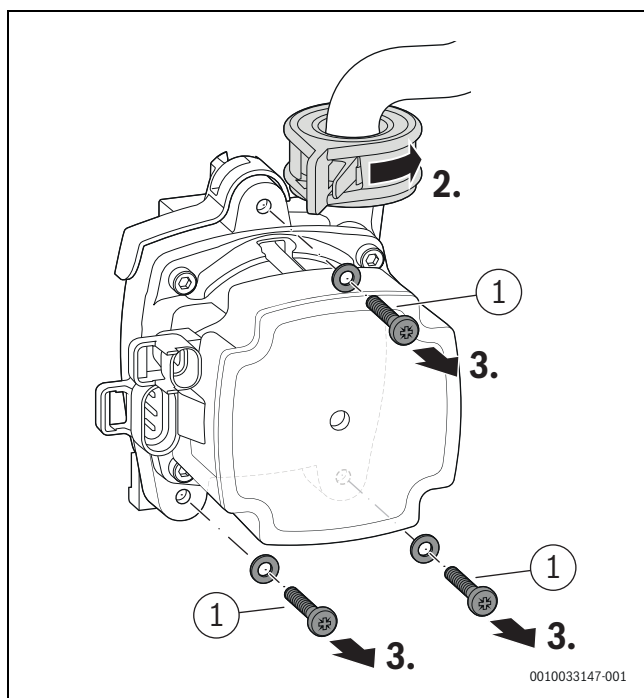
Rys. 142 Odblokowanie pompy c.o. i usuwanie śrub
