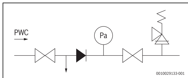
Rys. 74 Przykład: grupa bezpieczeństwa w wody w zespole rozprężnym wg EN 1488
