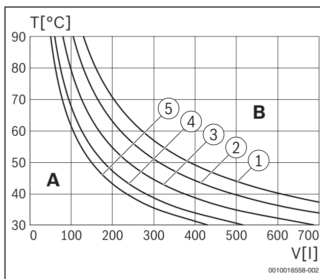
Rys. 46 Krzywe charakterystyki naczynia wzbiorczego (12 l)
