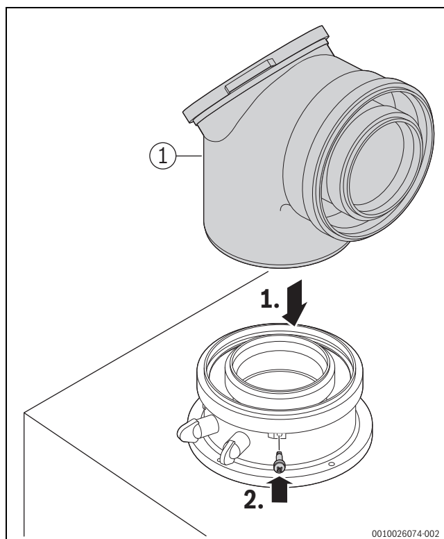
Rys. 79 Wkładanie osprzętu spalinowego i zabezpieczenie go śrubą
