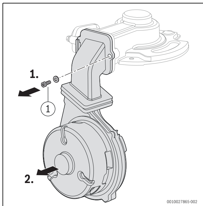
Rys. 128 Demontaż wentylatora i zespołu mieszającego
