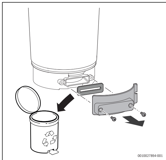
Rys. 136 Otwieranie otworu kontrolnego
