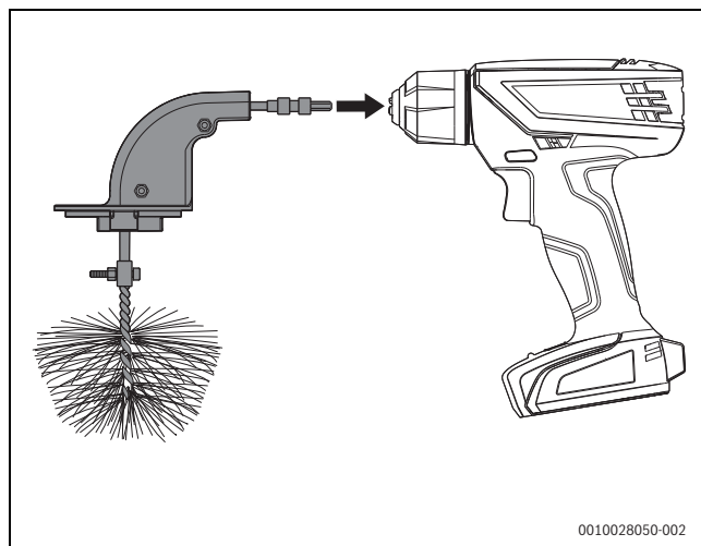
Rys. 134 Łączenie szczotki z wkrętką akumulatorową
