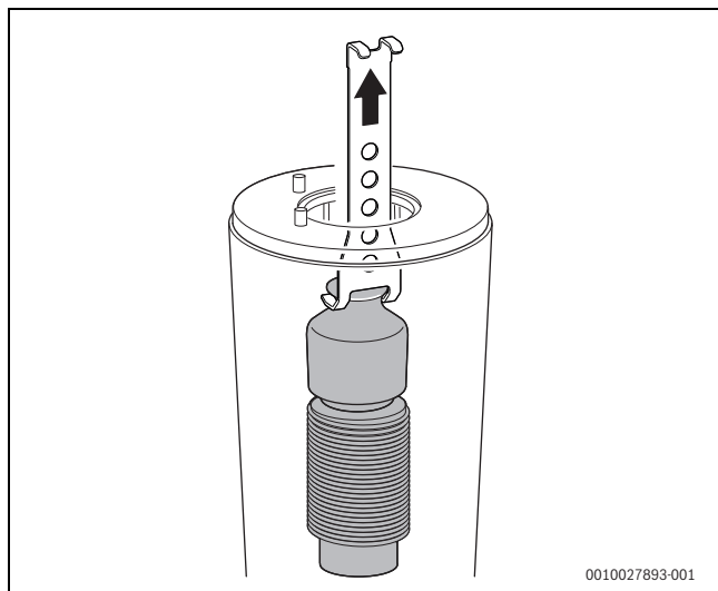
Rys. 131 Wyjmowanie górnego elementu wyporowego
