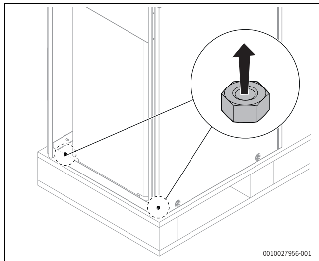
Rys. 49 Usuwanie zabezpieczenia transportowego na dole w tylnej części zasobnika
