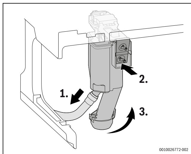
Rys. 154 Demontaż syfonu kondensatu
